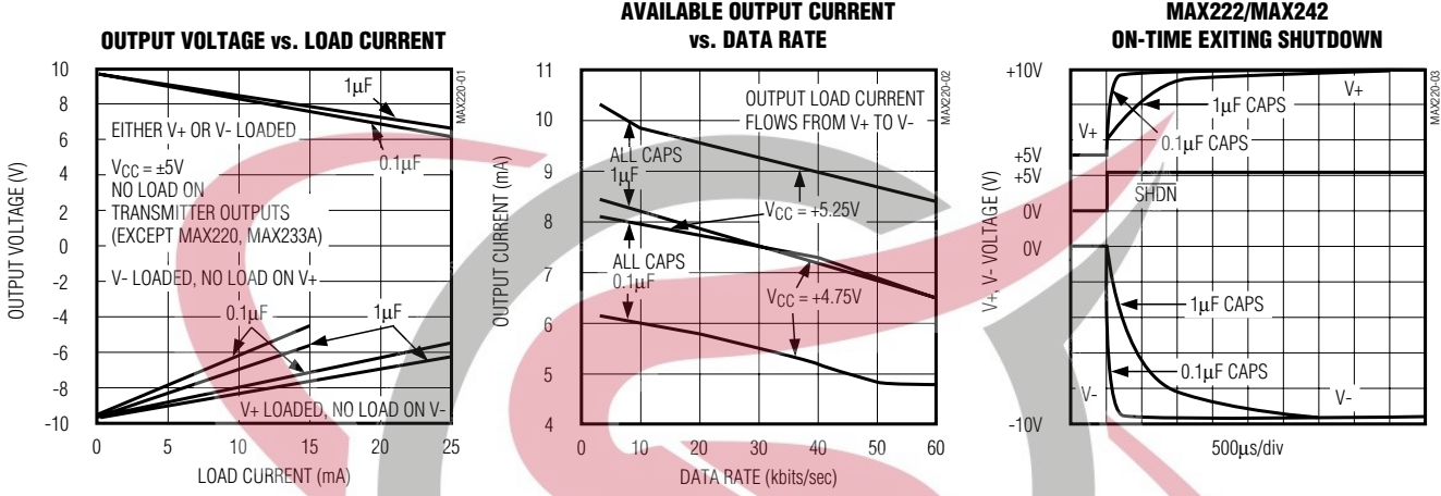
MAX220/MAX222/MAX232A/MAX233A/MAX242/MAX243
